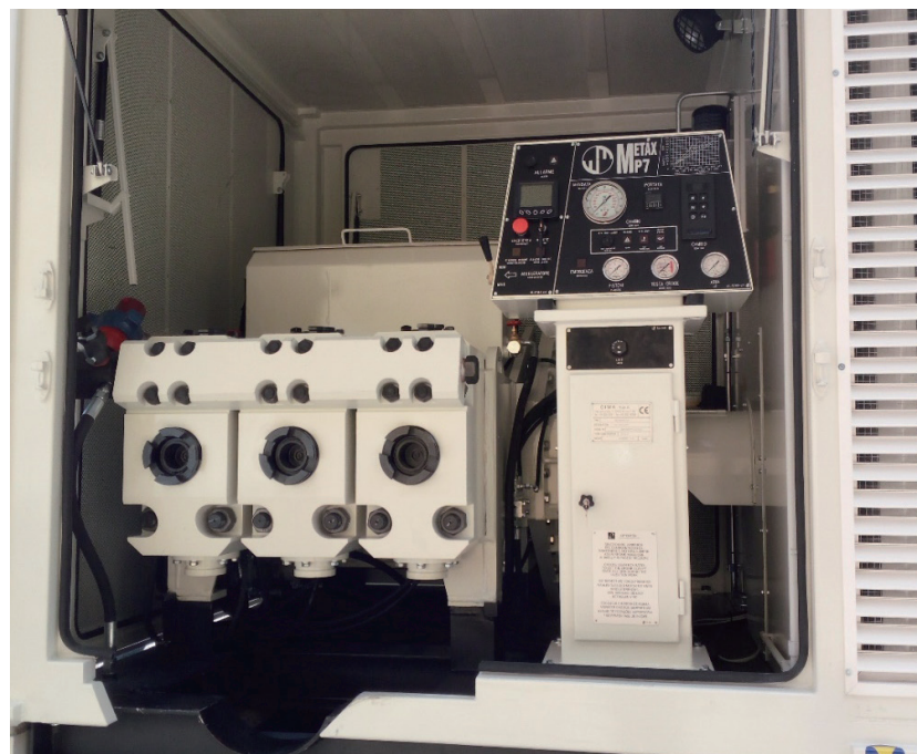
トリプレックスポンプ 操作盤
